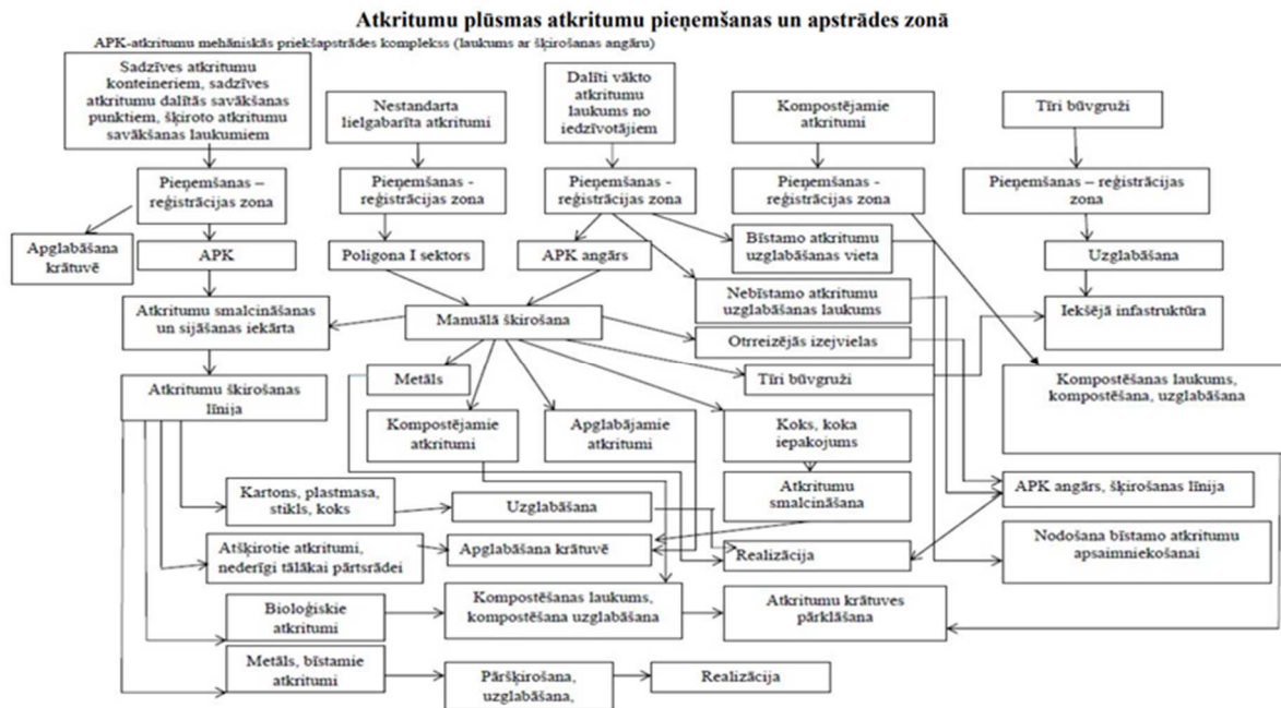
Attēls 7. Atkritumu plūsmas atkritumu poligonā "Kaudzītes"
