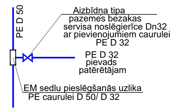
Mezгла ŪM-2, ŪM-3, ŪM-4, ŪM-5, ŪM-6, ŪM-7, ŪM-8 shēma
